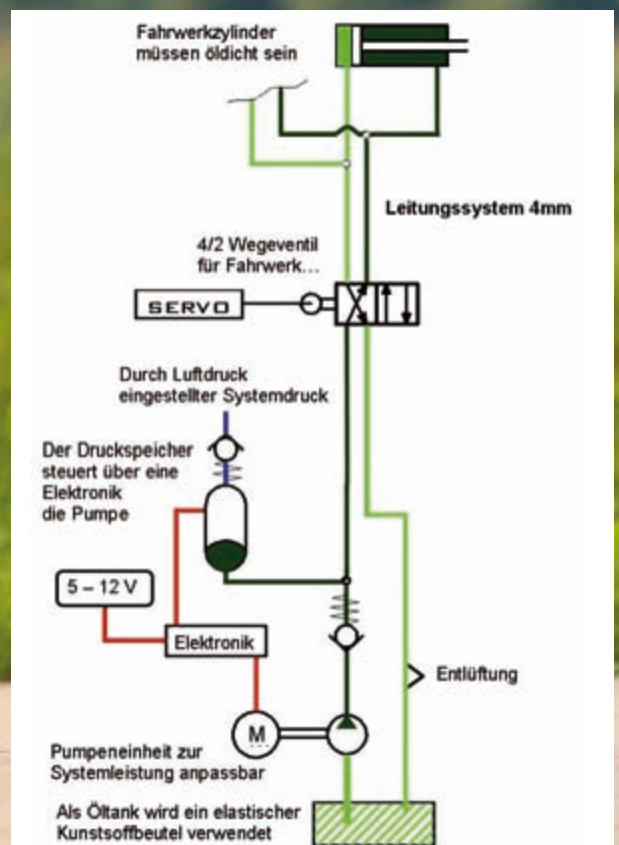
Systemdarstellung der Hydraulikanlage
